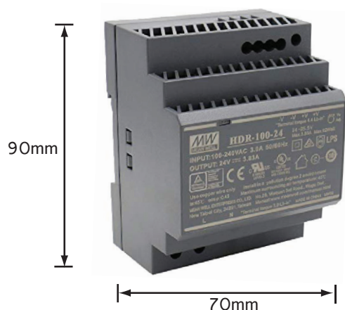
尺寸：70 (W) x 90 (H) x 54.5 (D) mm
