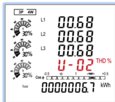
螢幕顯示範例一 查看電壓分次諧波
